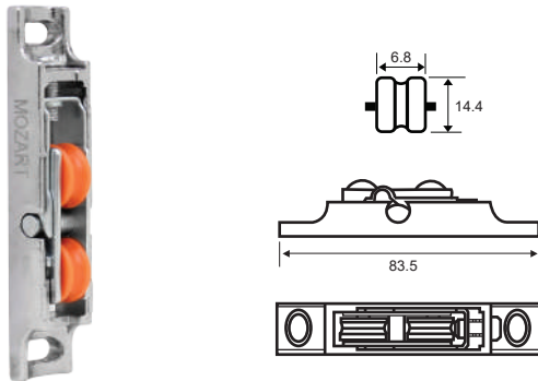
● Mini Adjustable Nylon Double Roller Code - MOZ 1752
